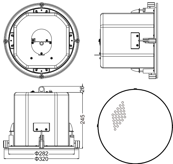
Measurement尺寸 (Unit单位: mm毫米)
